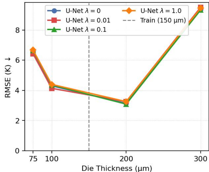
OOD: Die Thickness
